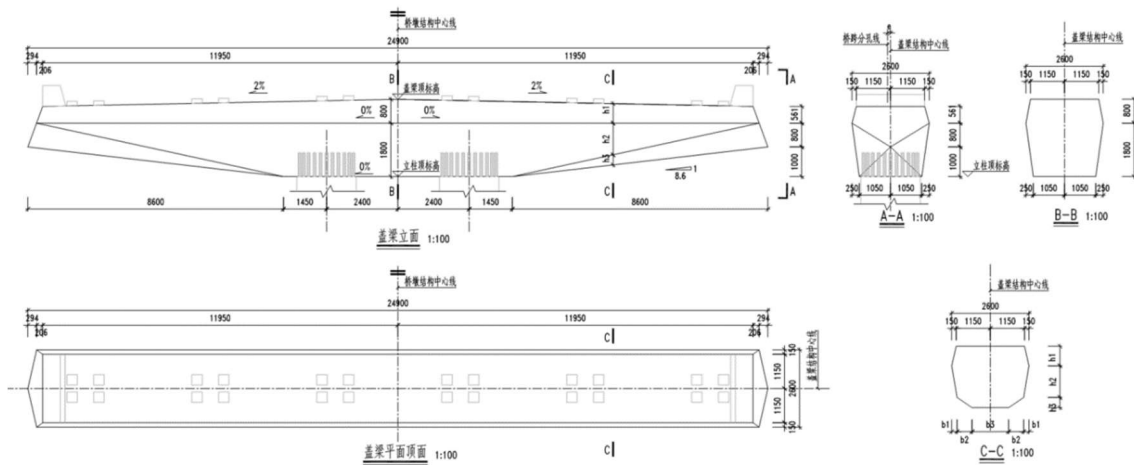
图 1.1-1 GL1、GL2 型盖梁施工图
