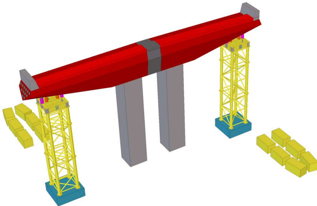
图 2.1-2 不落地支撑设计概念图
