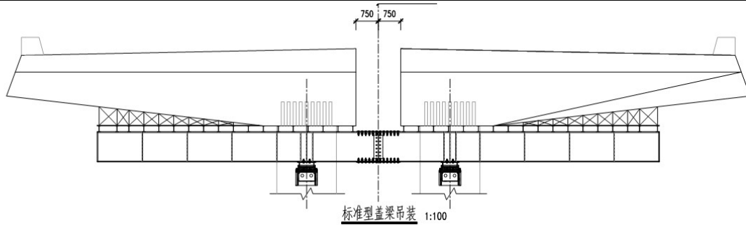
图 2.1-1 不落地支撑设计概念图
